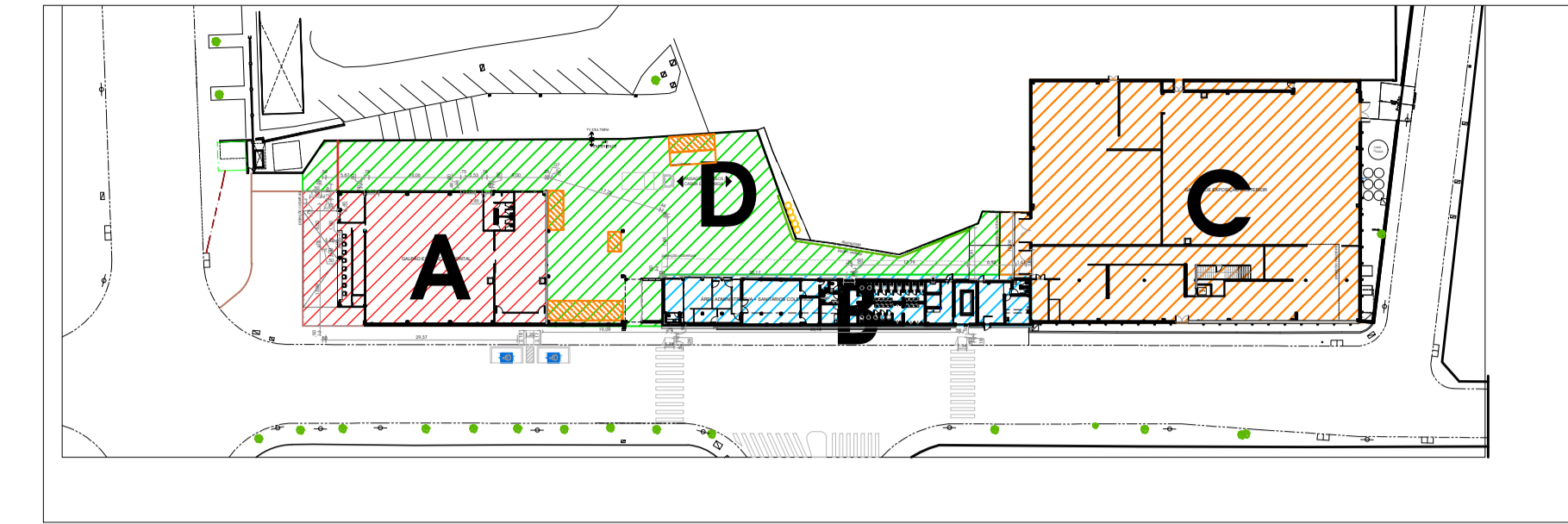
PLANTA DE SETORIZAÇÃO ESC. 1:250
