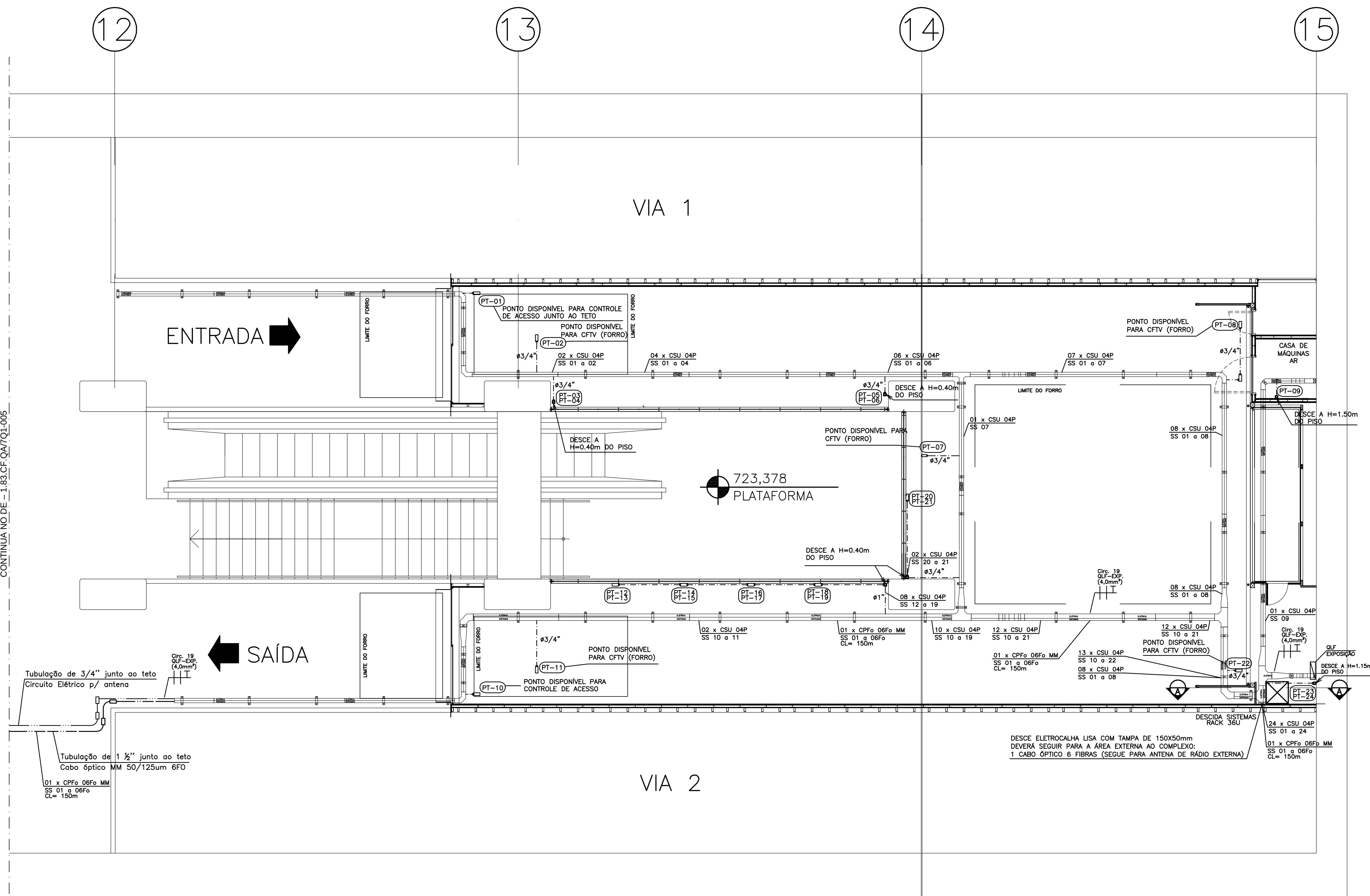
PLANTA_BAIXA ESCALA_1:50
