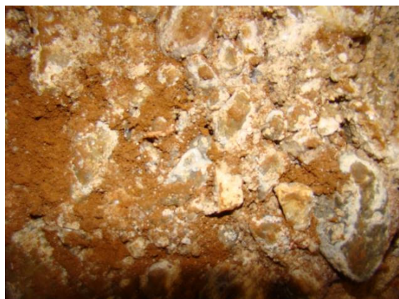
Prospecção Arquitetônica mostrando a composição dos materiais da fundação, com pedras e cimento
