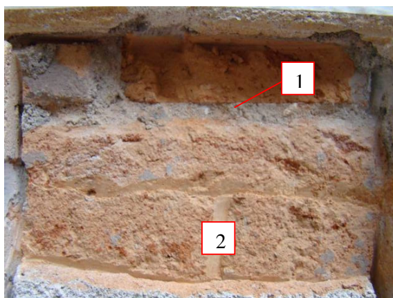
Detalhe do método construtivo em tijolos de barro (2) assentado com argamassa de areia e cal (1)
